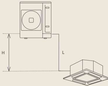
Configuración split individual (de 3 a 6 HP)
