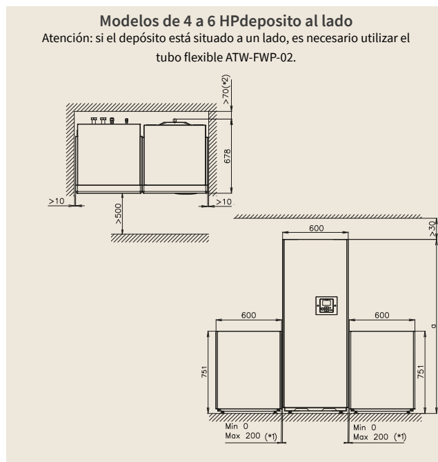
Dimensiones según el modelo (mm) - depósito en el lateral
