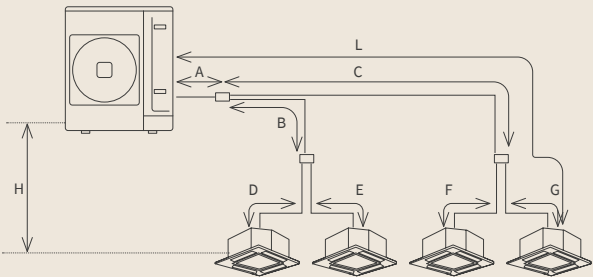
Configuración QUADRI (de 4 a 6 HP)
