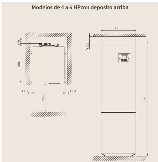
Dimensiones según el modelo (mm) - depósito en la parte superior
