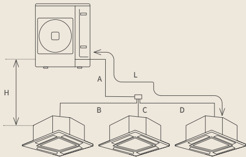
Configuración TRIPLE (de 4 a 6 HP)
