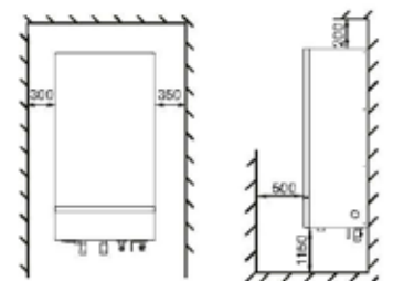
Espacio instalación
